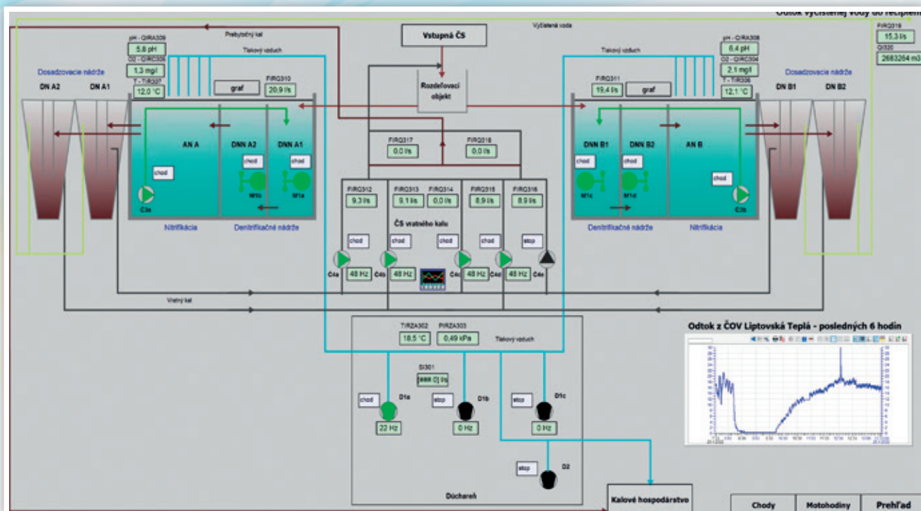
Dispečingový systém – Bloková schéma ČOV L. Teplá
