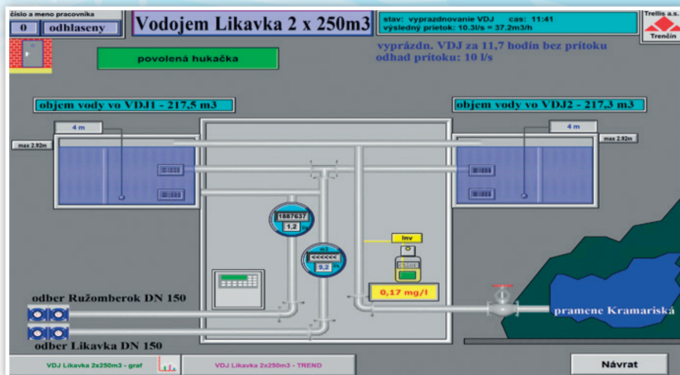
Dispečingový systém – Bloková schéma VDJ Likavka (2x500m³)
